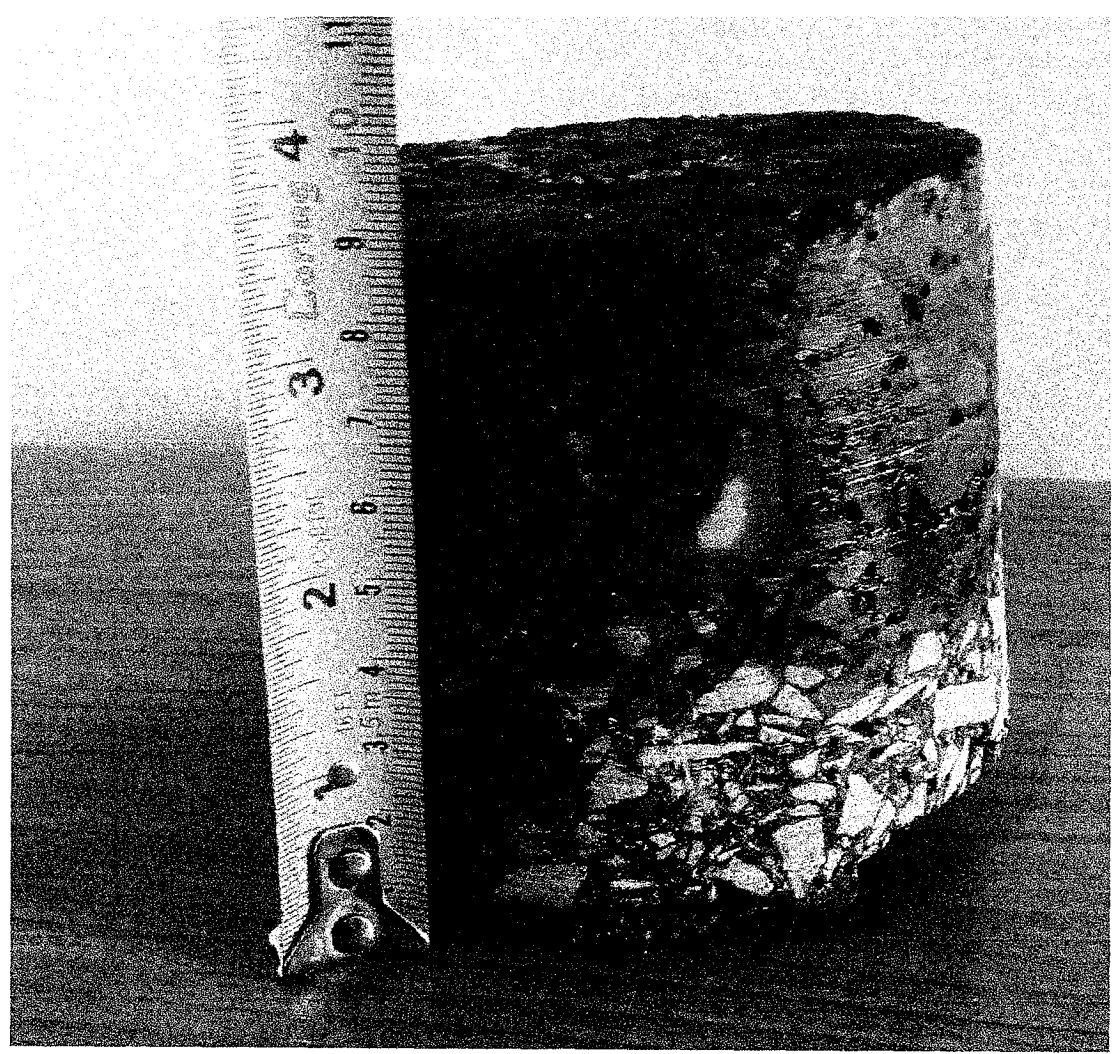
FIGURA 14: AMOSTRA 02 – F2.
