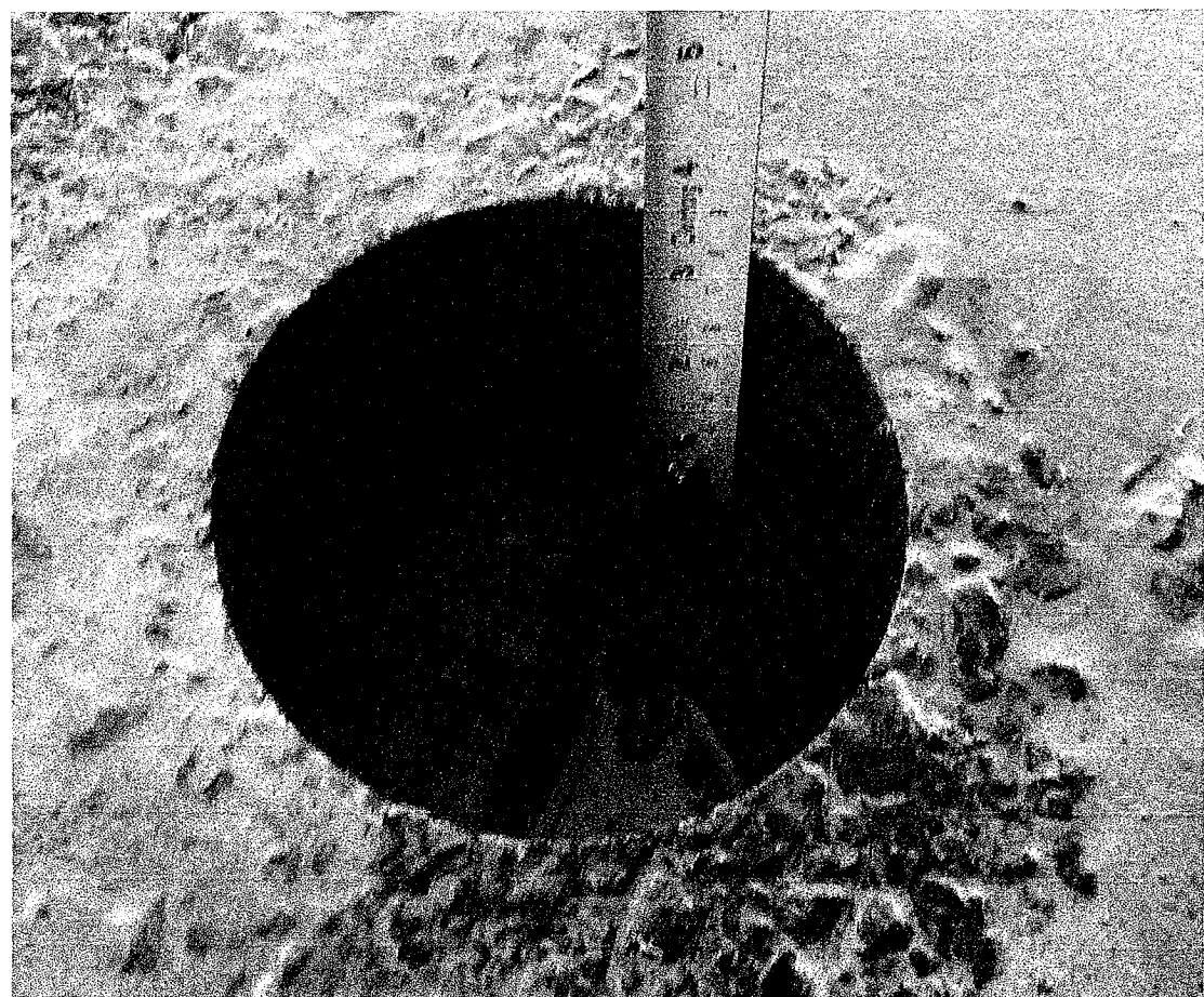
FIGURA 6: FURO 06 – F3.
